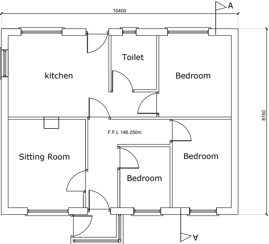
PLAN SCALE; 1:100
