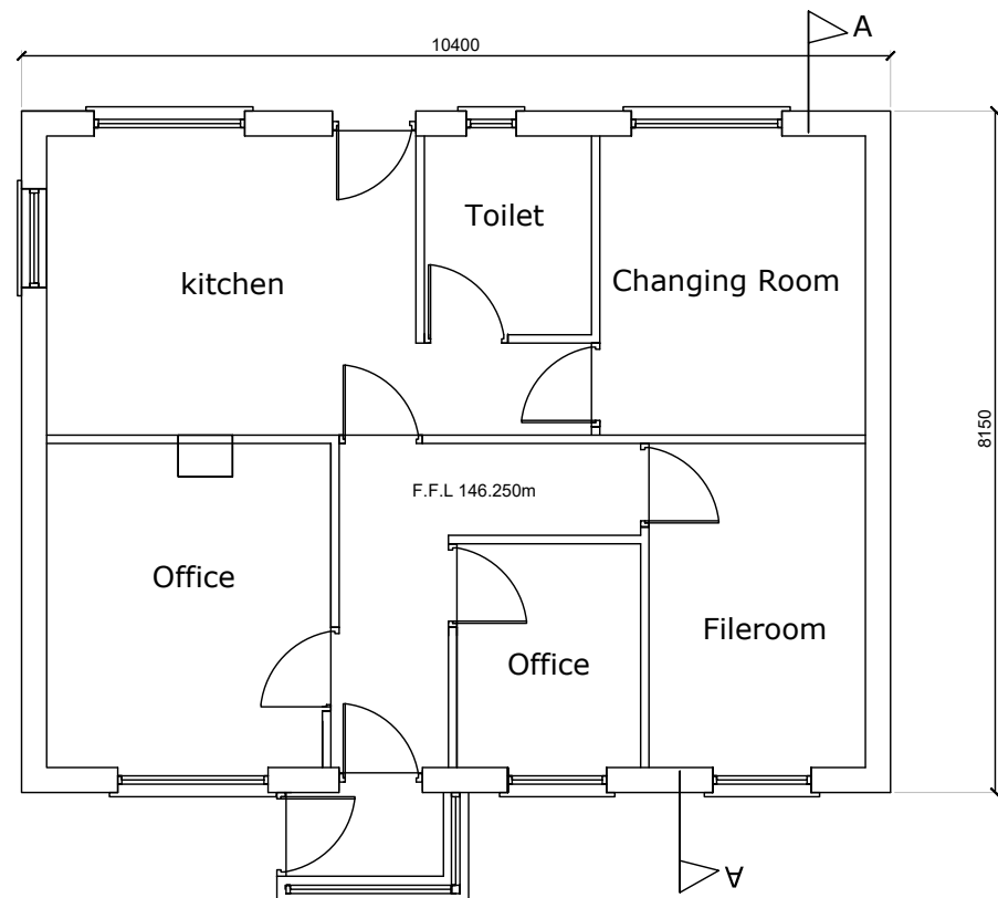
PLAN SCALE; 1:100
